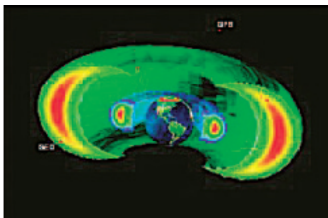
図1：地球をとりまく放射線帯 地球近傍の内帯とその外側にある外帯に分かれている (NASA TM 2002.2116.13)
