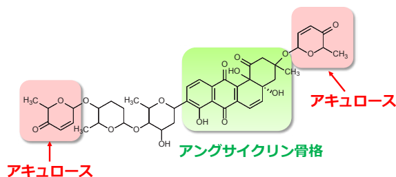
図.2 サブロルマイシン E の構造
