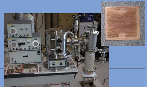
木質炭素素材でできた高機能DLC膜を 作製するための装置と得られたサンプル Apparatus for coating DLC film of carbonized wood with high functions and image of the obtained sample
