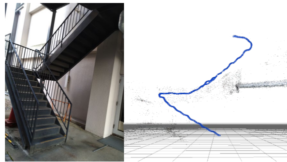
フォトグラメトリ解析による3次元歩行解析
