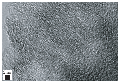
図2-2：600℃で熱処理した主としてミクロ孔からなる木質炭素の電子顕微鏡図
