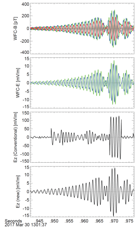
図1：電界波形の未計測成分推定
