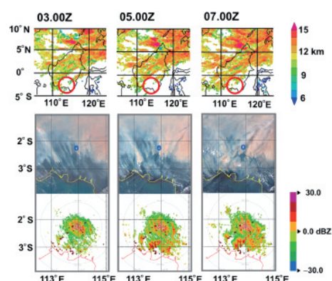
下から2015年10月15日03UT、05UT、07UTに気象レーダーで観測されたエコー強度分布、ひまわり衛星画像、雲頂高度。(Rahman et al., 2021)。
