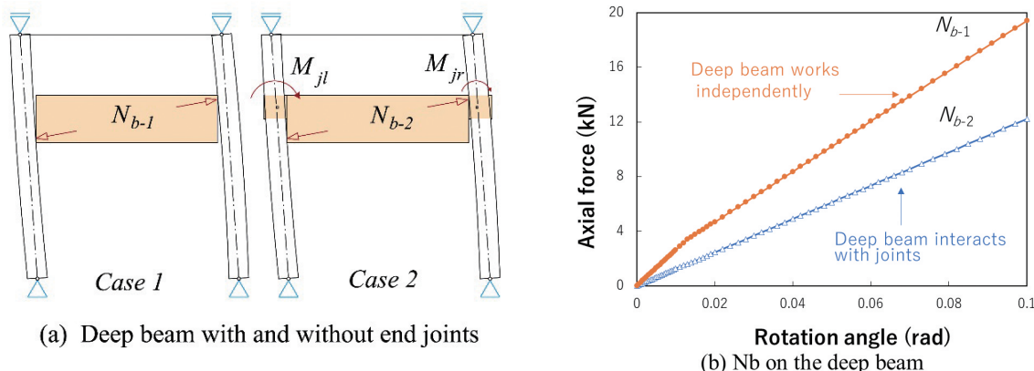
図2：差し鴨居仕口のある場合の影響
