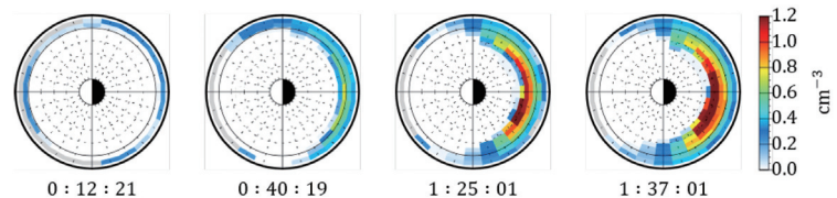
図3：移流シミュレーションで求めた南向き惑星間空間磁場期間における熱いH+イオンの密度
