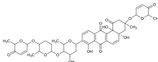
図. 2 サプロルマイシン E の構造
