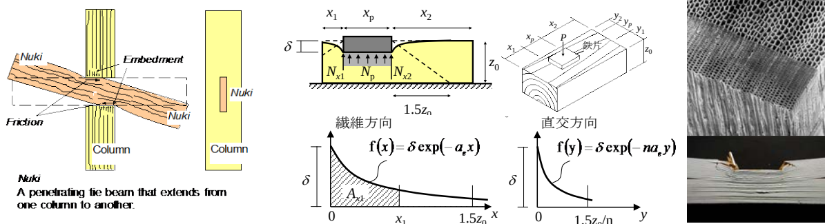
図5：貫接合部とめり込みの力学モデル 2)
