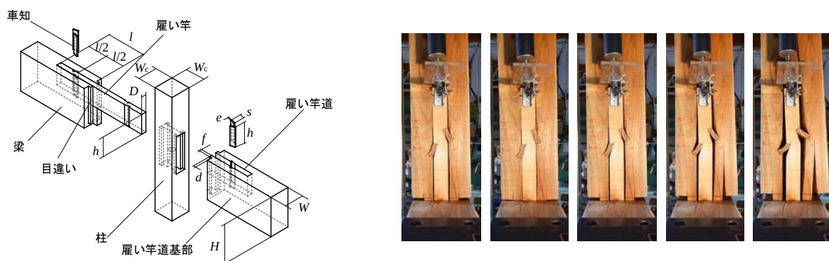
図6：雇い竿車知接合部と変形の様子
