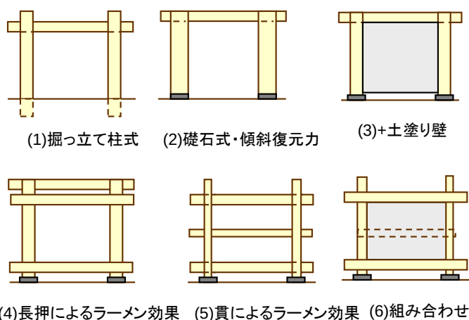
図 1：鉛直構面架構の分類
