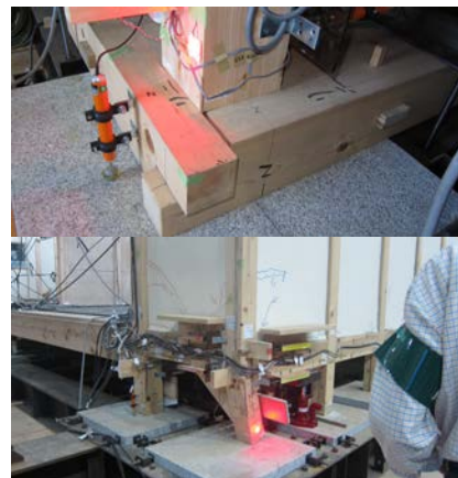
図 9：柱脚の足固めと柱の折損
