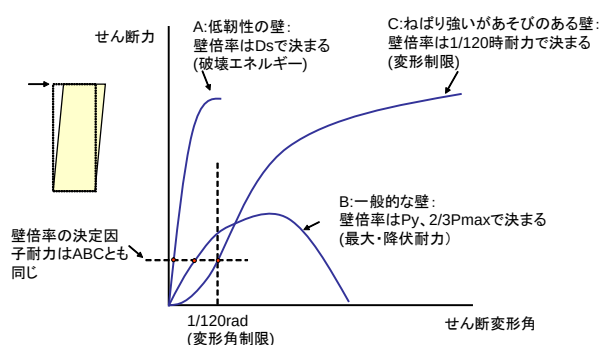
図 10：伝統木造住宅の地震被害と壁倍率の概念
