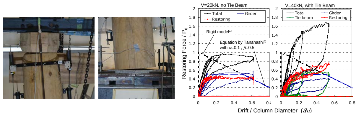
図8：柱復元力の実験例 9)
