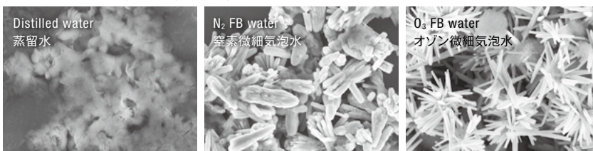
微細気泡の利用(無機化学) — 酸化亜鉛のSEM画像 Fine bubble applications (Chemistry) SEM images of ZnO
